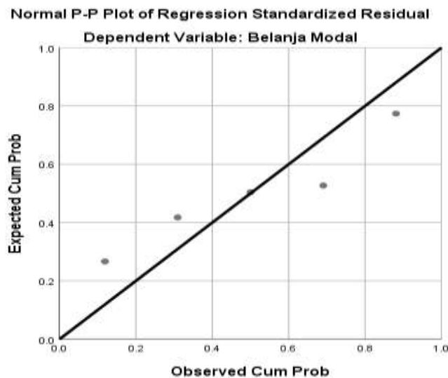
Gambar 4.1 Uji Normalitas
