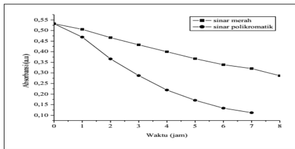
Gambar 8. Grafik kinetika degradasi klorofil daun Lamun dalam pelarut aseton selama 7 dan 8 jam iradiasi (pengukuran setiap 1 jam): (■) iradiasi dengan sinar merah, dan (●) iradiasi dengan sinar polikromatik
