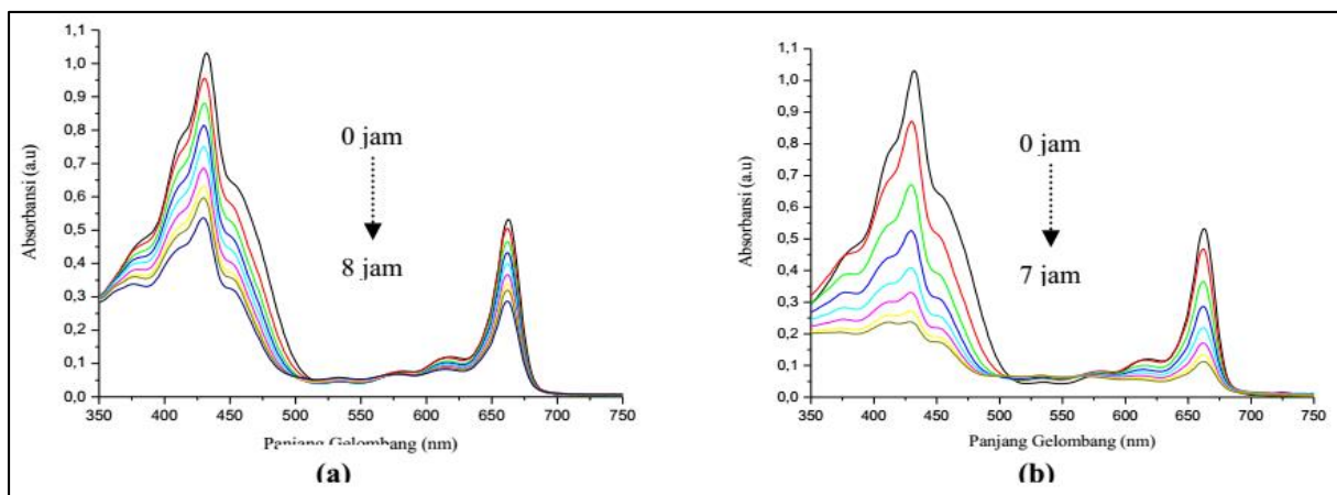
Gambar 5. Perubahan pola spektra absorpsi klorofil Lamun dalam pelarut aseton selama 8 dan 7 jam (pengukuran setiap 1 jam): (a) iradiasi sinar merah, (b) iradiasi sinar polikromatik
