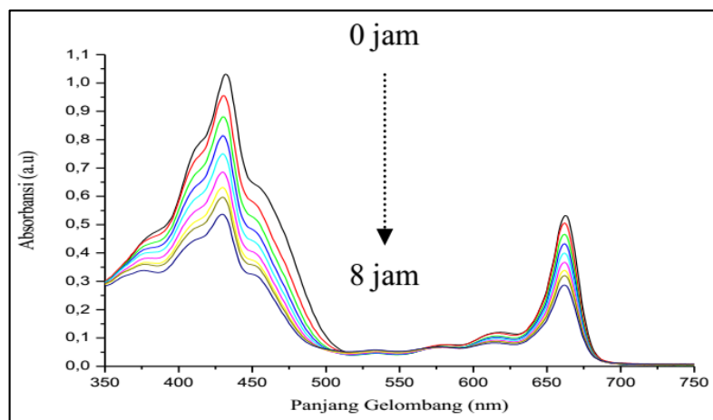
Gambar 4. Perubahan pola spektra absorpsi klorofil Lamun dalam pelarut aseton selama 8 jam iradiasi sinar merah (pengukuran setiap 1 jam)
