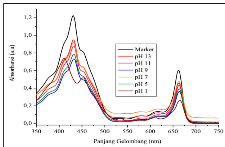
Gambar 3. Pola spektra norbixin dalam aseton dengan berbagai pH: pH 13(merah), pH 11 (hijau), pH 9 (biru), pH 7 (orange), pH 5 (olive) dan pH 1 (wine)
