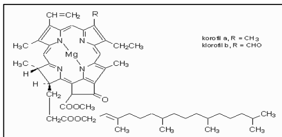
Gambar 1. Struktur senyawa kimia klorofil dengan inti atom Magnesium (Mg)
