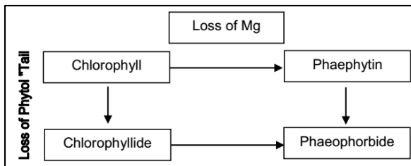
Gambar 2. Bagan proses degradasi klorofil menjadi turunannya
