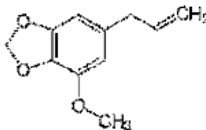
Gambar 1. Struktur kimia miristisin
